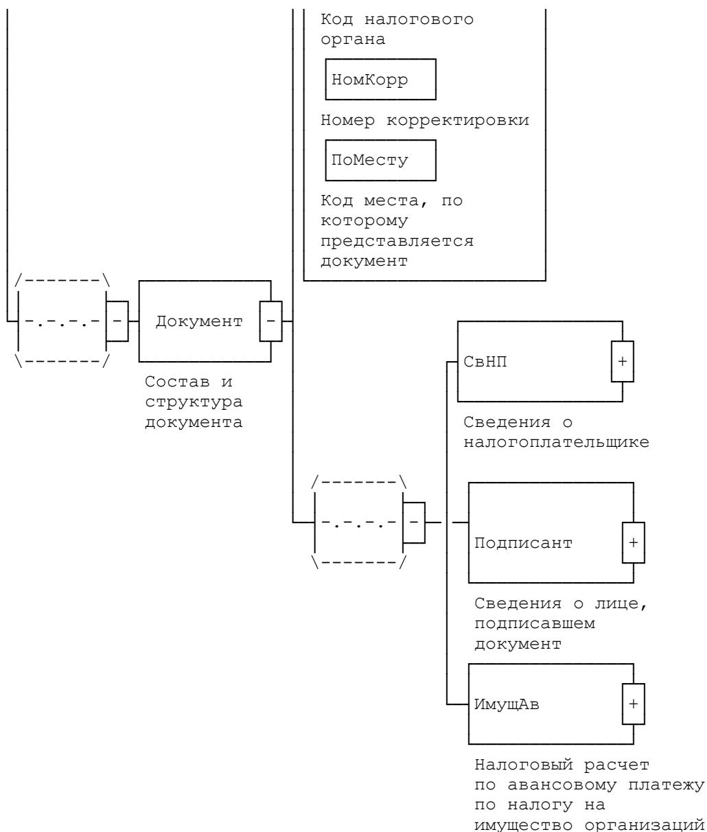
Рисунок 1. Диаграмма структуры файла обмена
